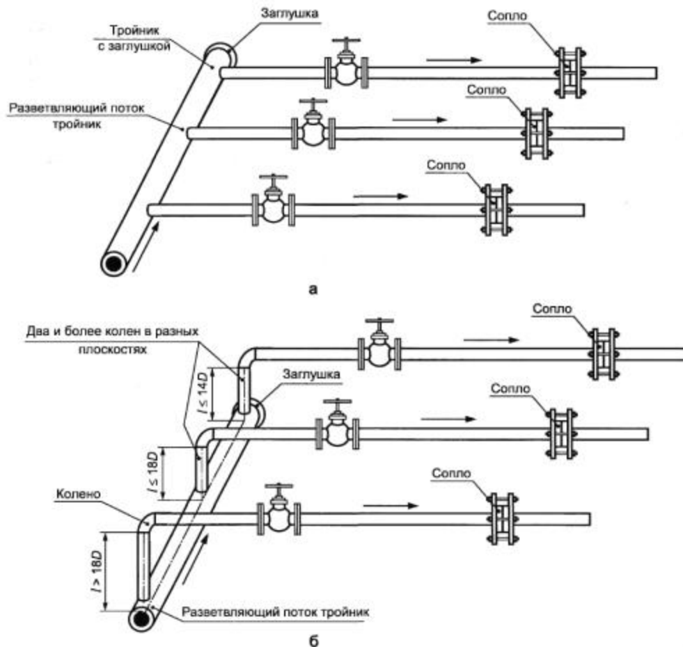
Рисунок 5 - Схемы коллектора
