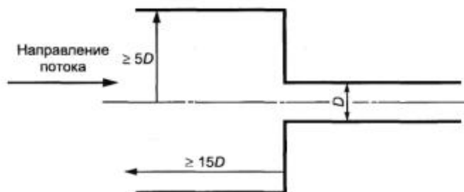
Рисунок А.5 - Схема большой емкости
