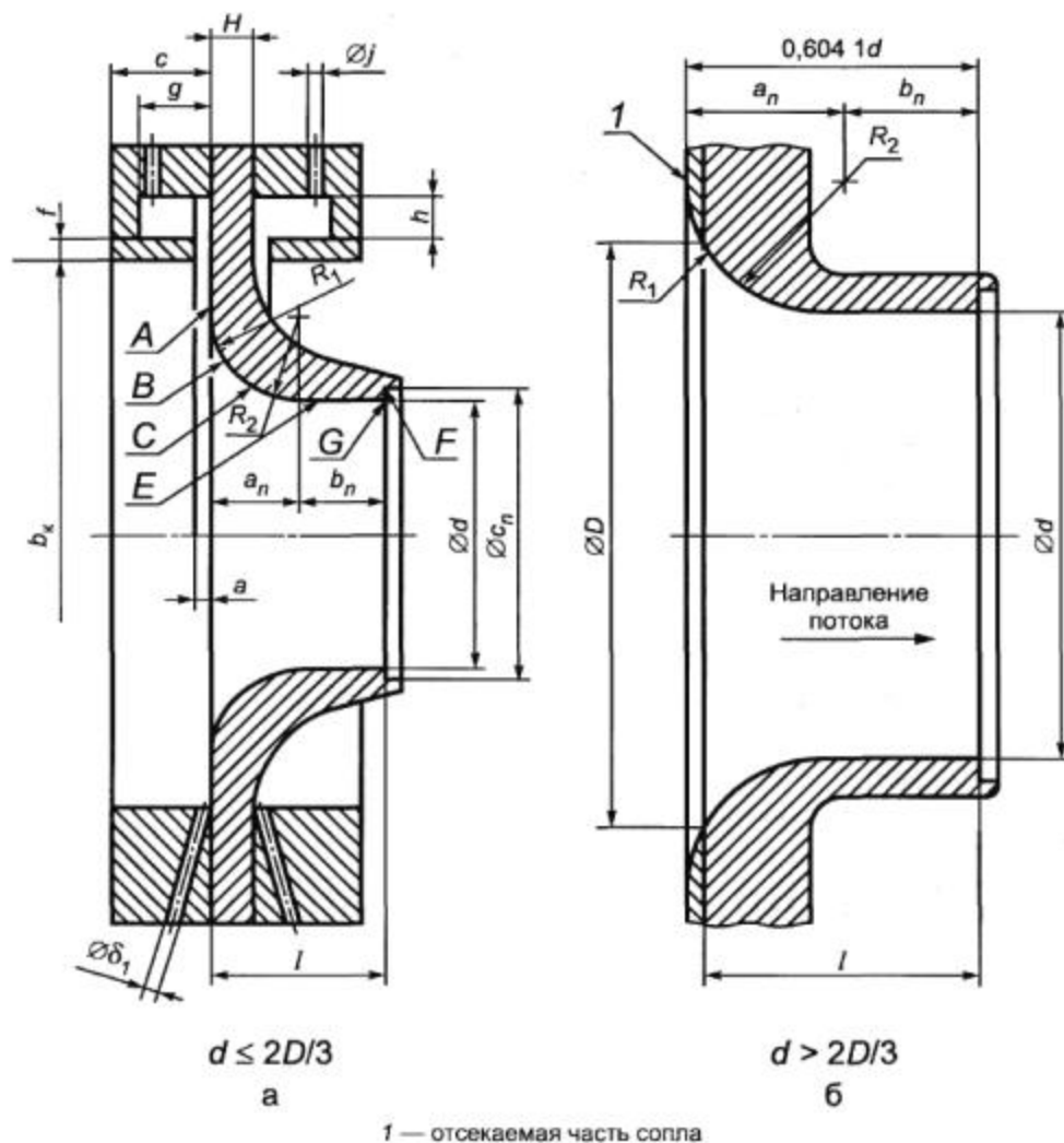
Рисунок 1 - Сопло ИСА 1932
