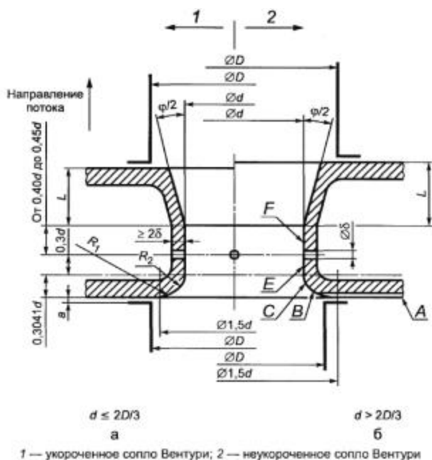
Рисунок 3 - Сопла Вентури
