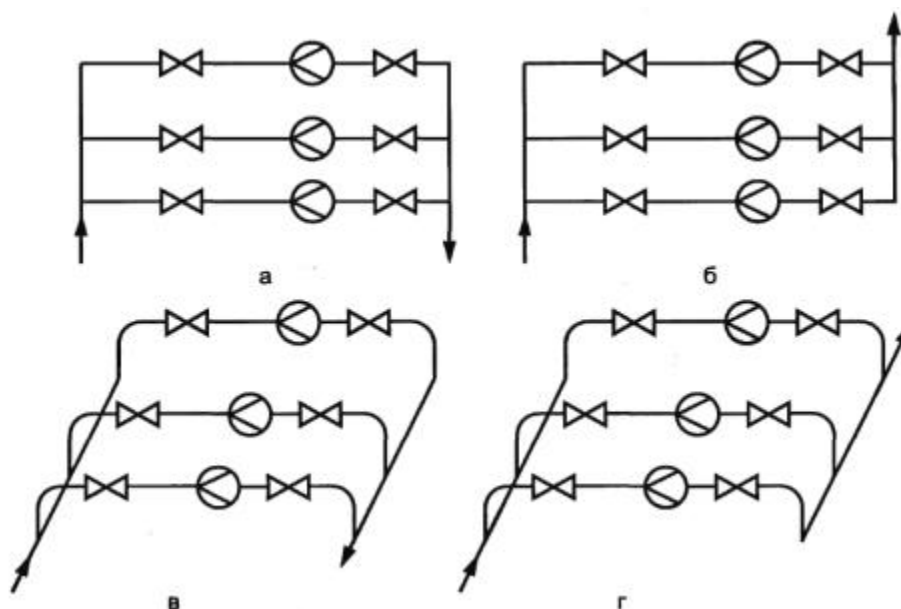
Рисунок А.4 - Схемы коллекторных систем
