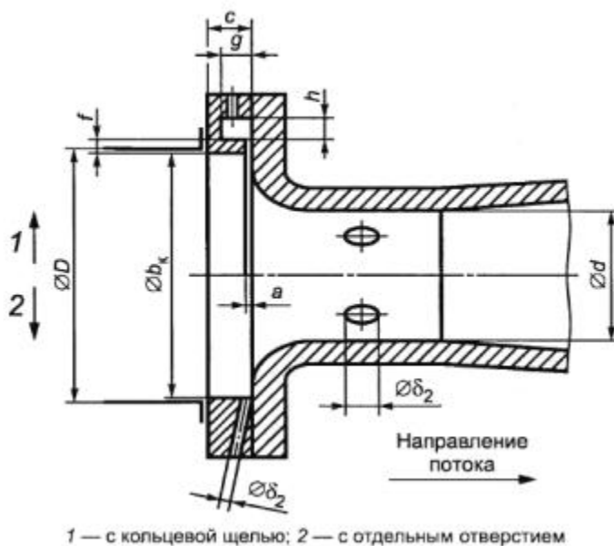
Рисунок 4 - Способы отбора давления, используемые для сопел Вентури
